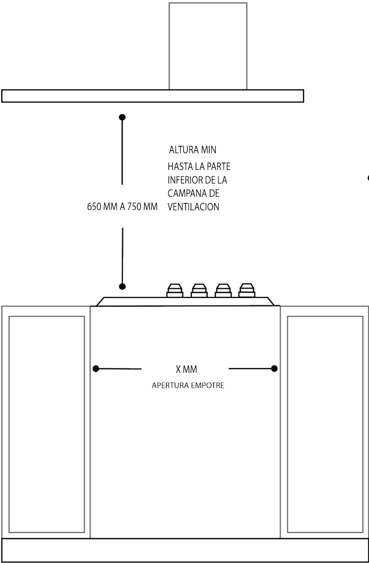
DISTANCIA PERMITIDA ENTRE PARRILLA Y CAMPANA
