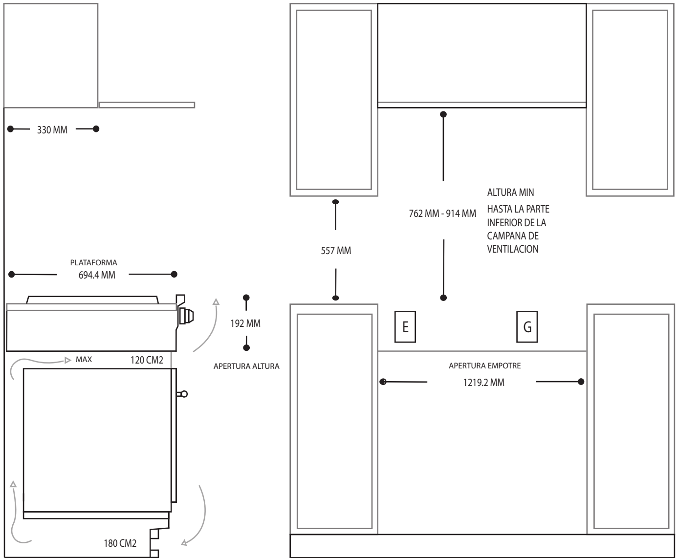
VISTA LATERAL
